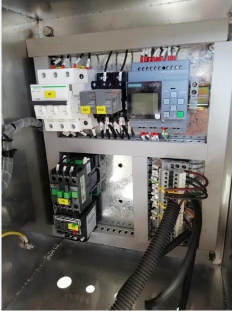
Control Cabinet: Schneider/Siemens
